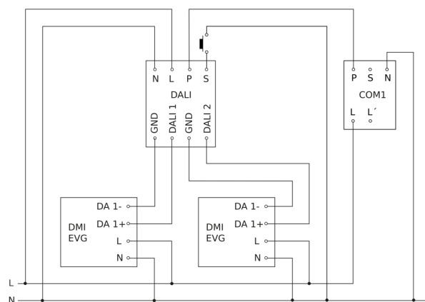
Schema elettrico Master-Slave collegamento in rete
